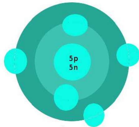
Boron 2,3
